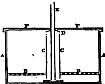
FIG. 3.—Section of Kier (old form).
